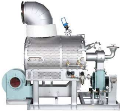
写真は、LNG 燃料船向けガス燃焼ユニット MECS-GCU (メックス ジーシーユー)
